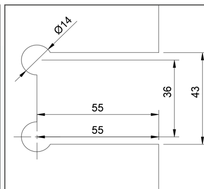
Tür ohne Dichtprofil (2 mm Spaltmaß)
