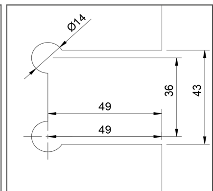
Tür mit Dichtprofil (8 mm Spaltmaß)
