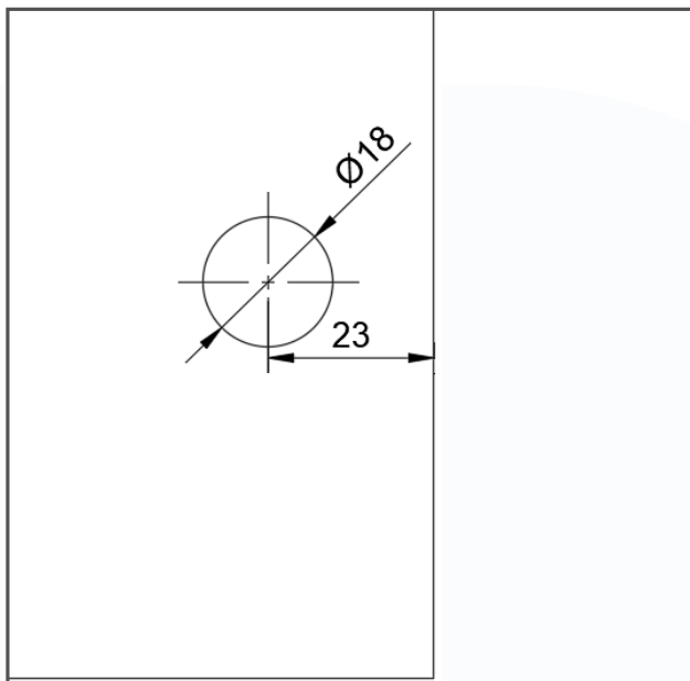
Festteil A (2 mm Spaltmaß)
