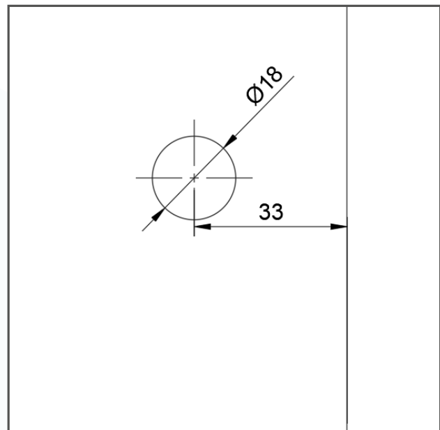
Festteil B (2 mm Spaltmaß)
