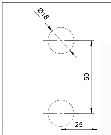
Festteil ohne Dichtprofil (2 mm Spaltmaß)
