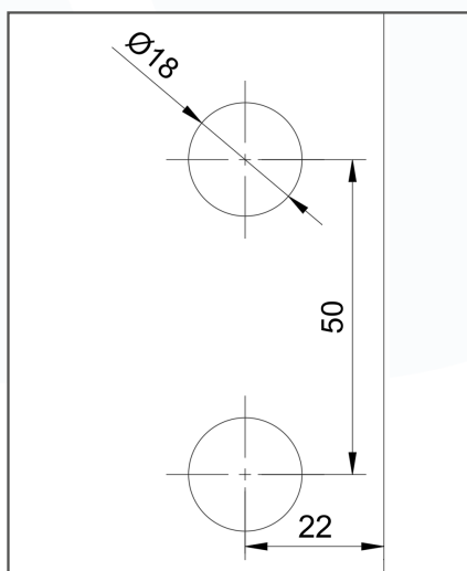
Festteil mit Dichtprofil (8 mm Spaltmaß)
