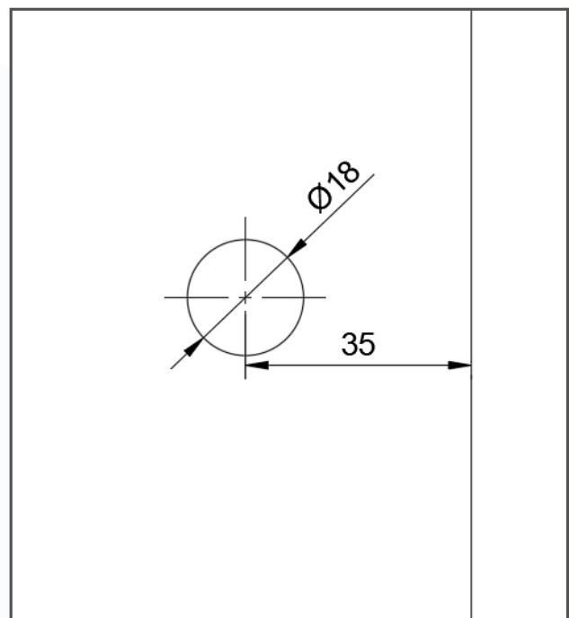
Festteil B (2 mm Spaltmaß)
