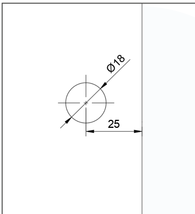
Festteil A (2 mm Spaltmaß)
