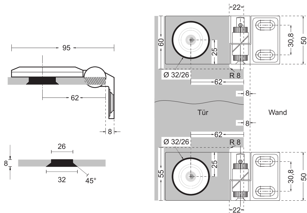
Zeichnung Ausschnitt für DIN links
